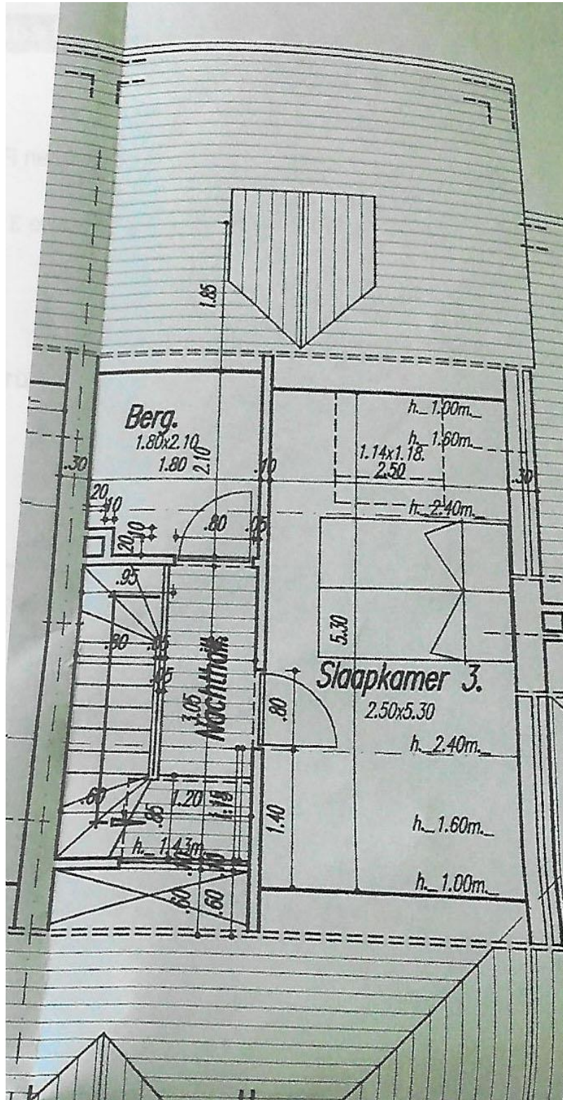
Woning 5 Veldstraat 10 3 de verdiep
