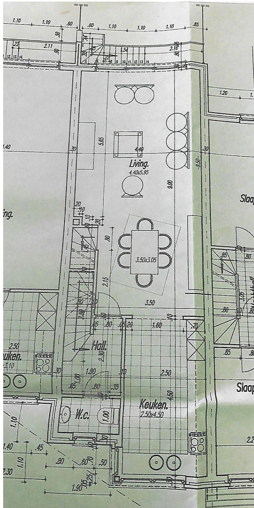
Woning 5 Veldstraat 10 1 ste verdiep
