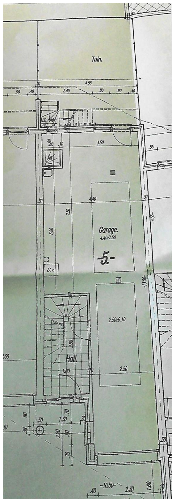
Woning 5 Veldstraat 10 Gelijkvloers
